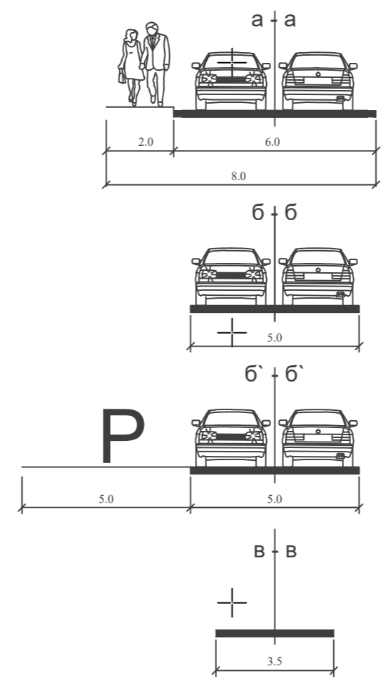
КАРАКТЕРИСТИЧНИ ПОПРЕЧНИ ПРОФИЛИ САОБРАЋАЈНИЦА
