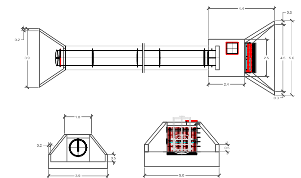
основа и изгледи пропуста
